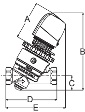
PCTVS15
